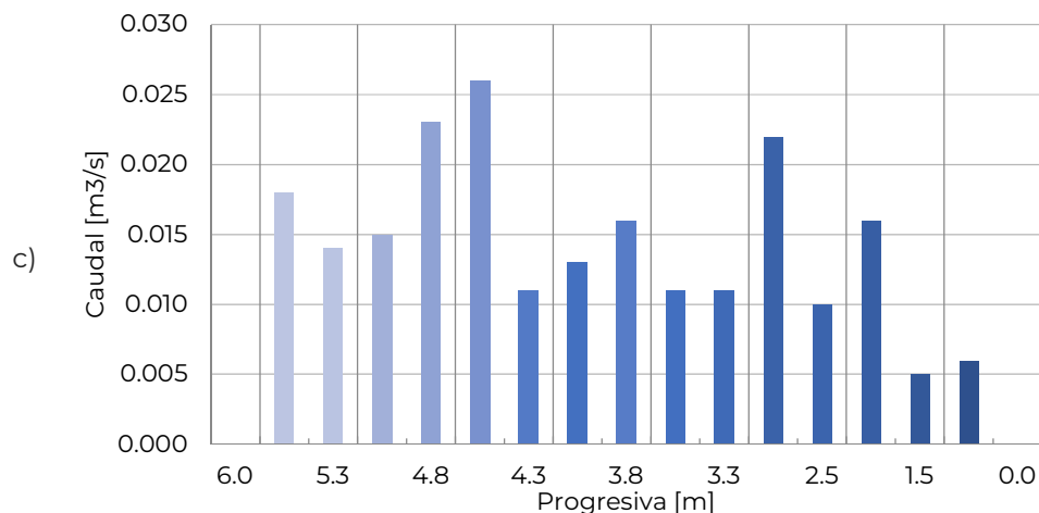
Figura 4. (a) Sección transversal del arroyo Las Mojarras en el sitio de medición (c) caudal aforado. La progresiva 0.00 corresponde con la margen izquierda
