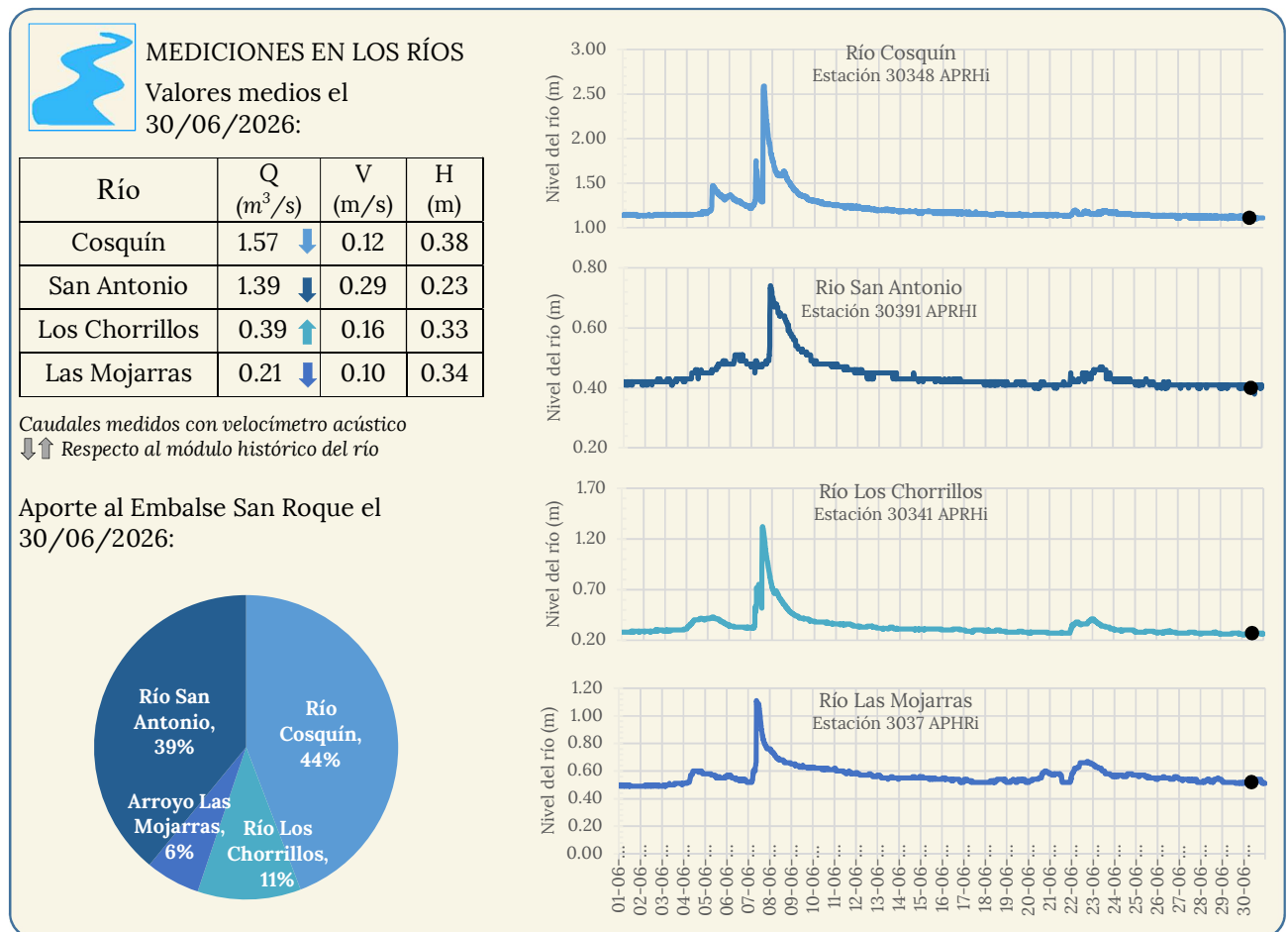
Figura 7. Resumen de las mediciones en los ríos el día 30/06/2026.
